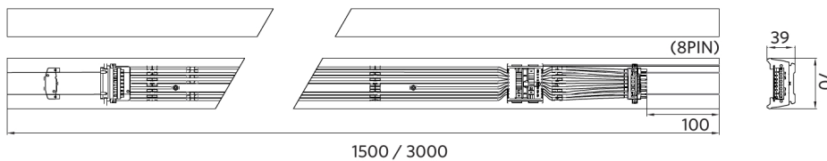
Tragschiene 8 Endstück
